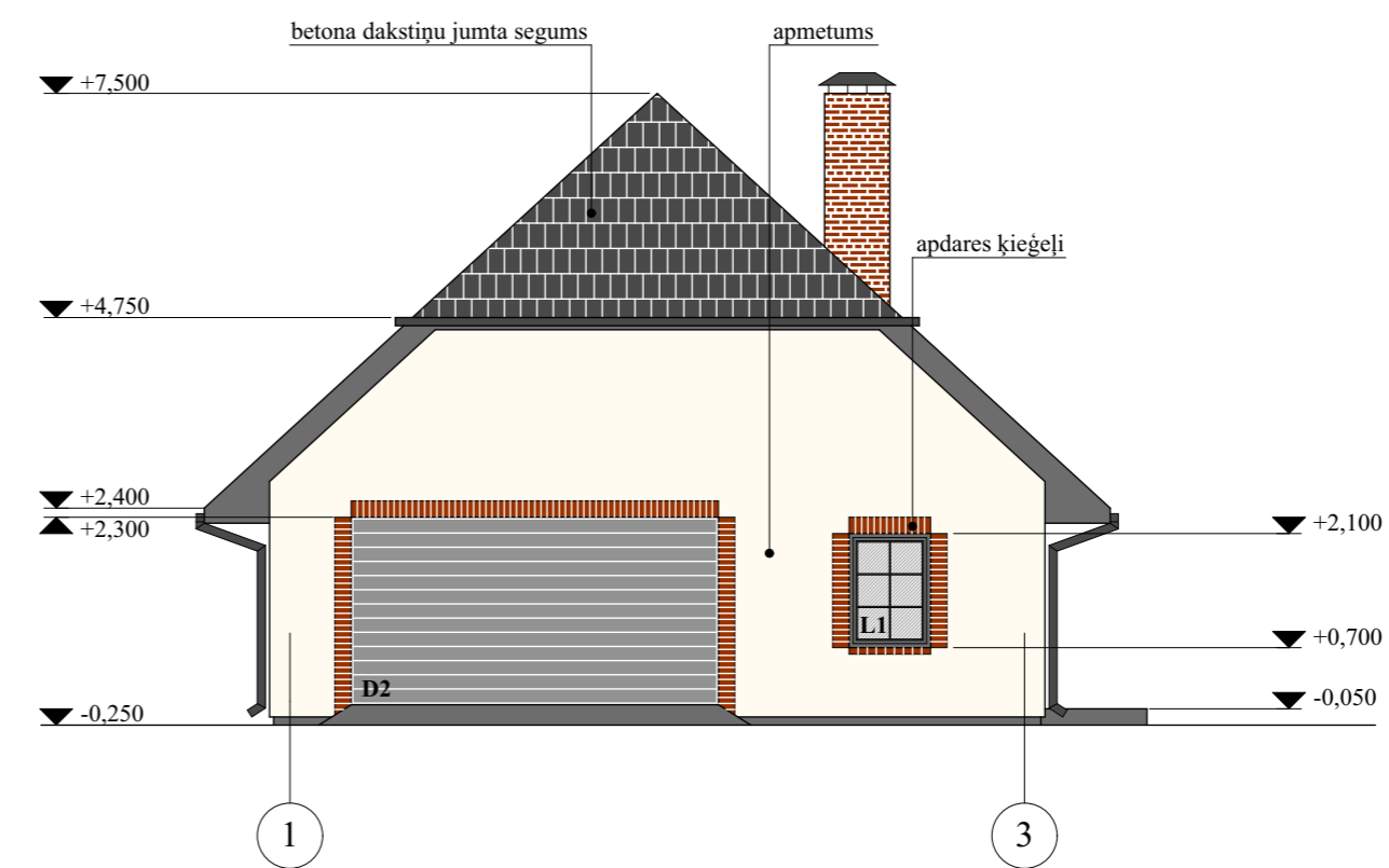
Fasāde asīs 1-3
