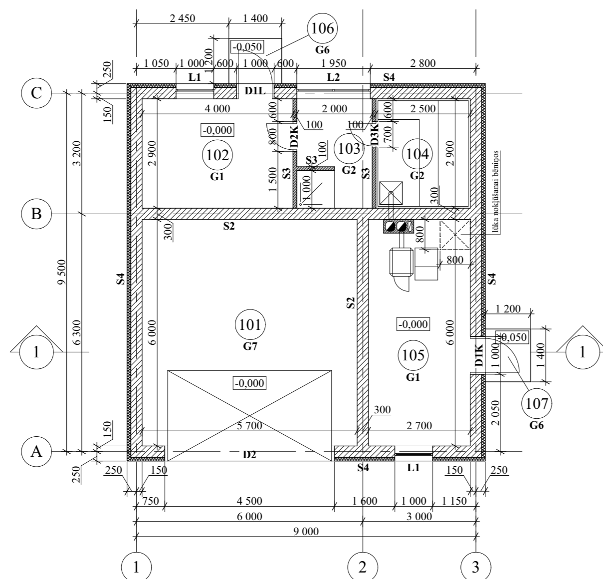
Garāžas plāns
