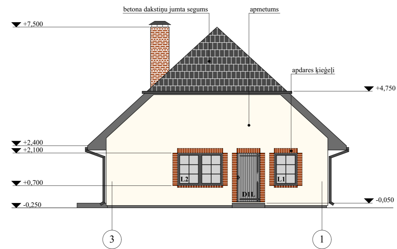
Fasāde asīs 3-1
