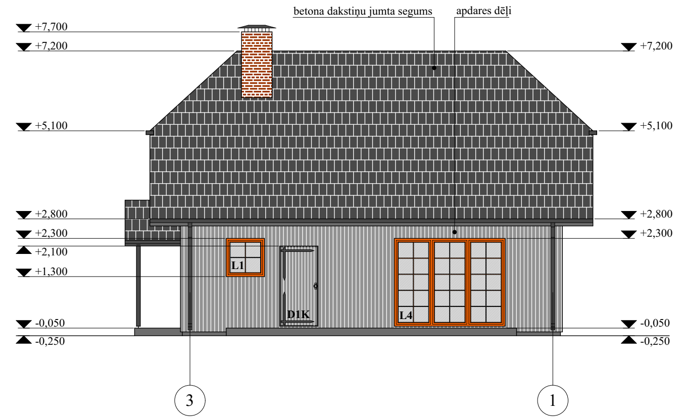
Fasāde asīs 3-1
