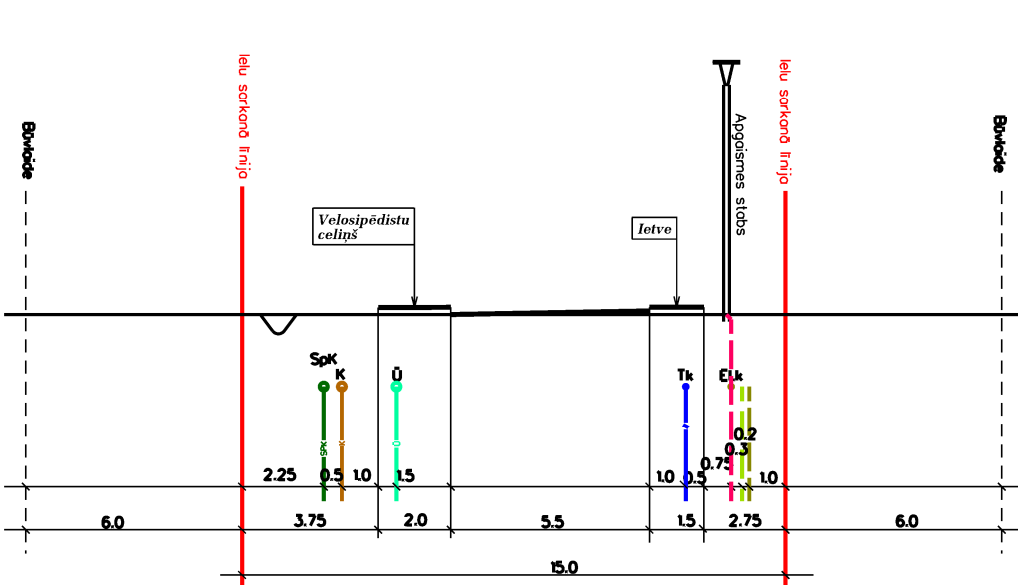
Projektējamās ielas šķēršprofils 2-2 M 1:300
