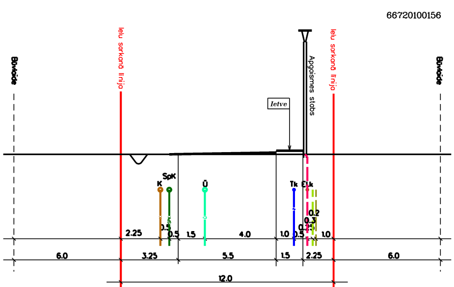
Projektējamās ielas šķēršprofils 1-1 M 1:300
